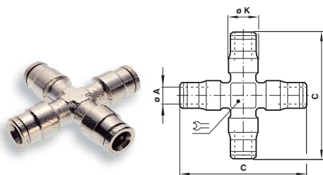
Raccordo a croce
