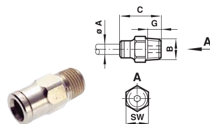
Raccorderia a tenuta
