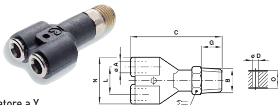
Adattatore a Y
