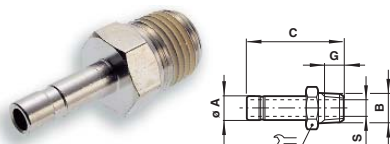
Raccordo diritto a codolo
