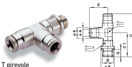
Raccordo laterale a T girevole
