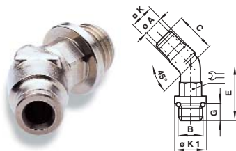
Adattatore girevole a 45°
