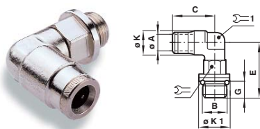
Gomito girevole a 90°
