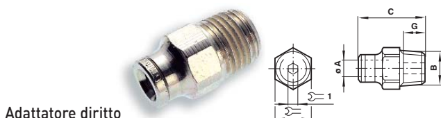
Adattatore diritto
