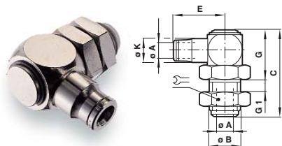
Raccordo passaparete a gomito girevole
